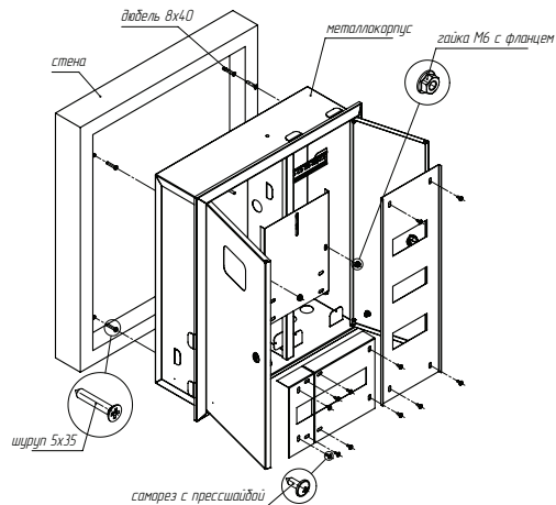
Рис. 1 - Схема монтажа
