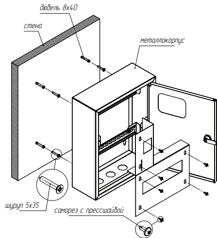
Рис. 1 - Схема монтажа
