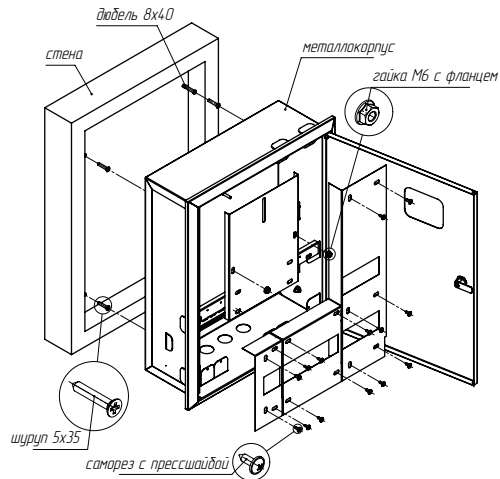
Рис. 1 - Схема монтажа
